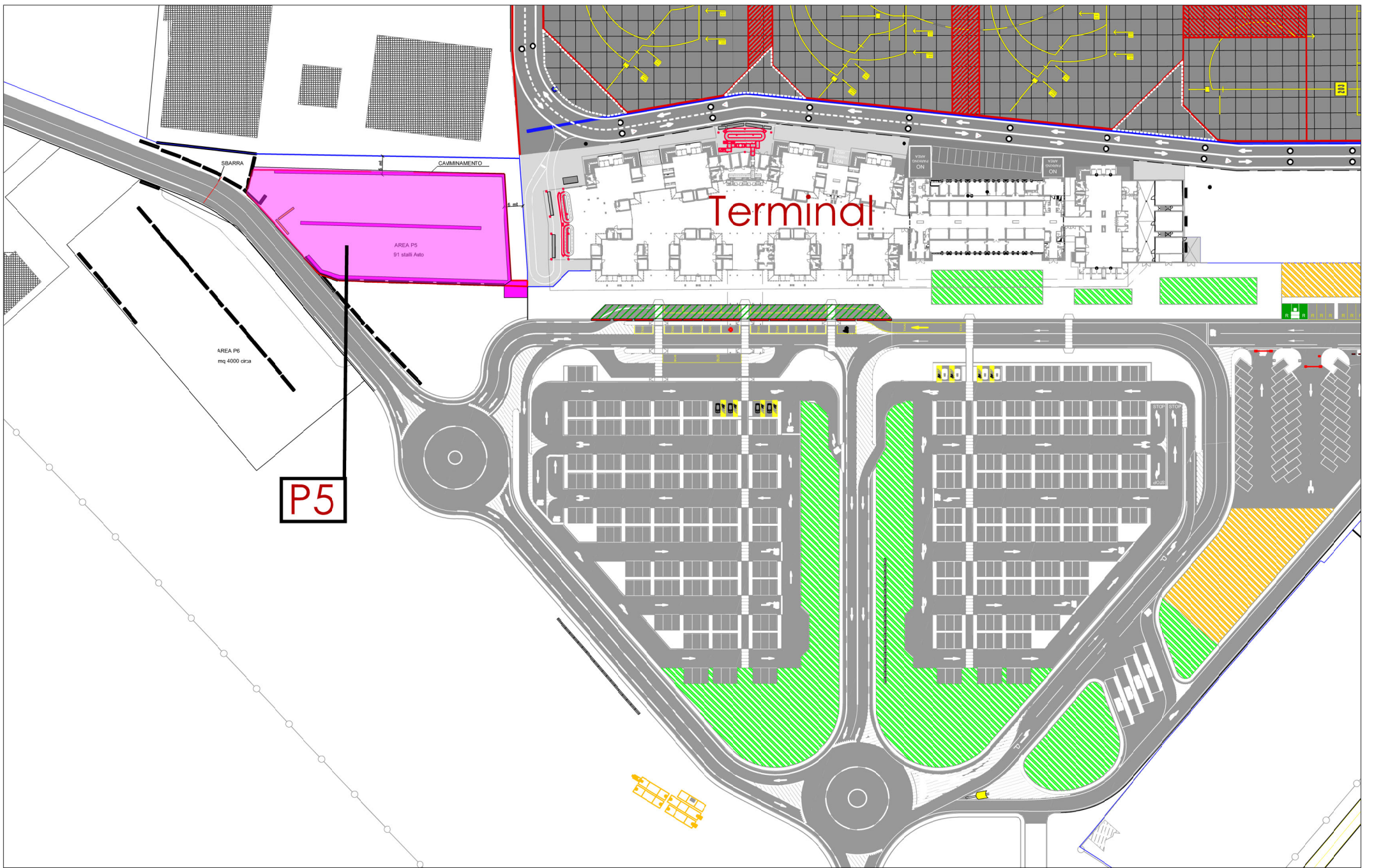
UBICAZIONE PARCHEGGIO P5
